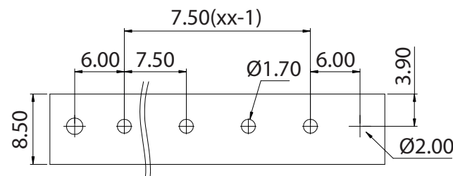
p.c.b. layout
