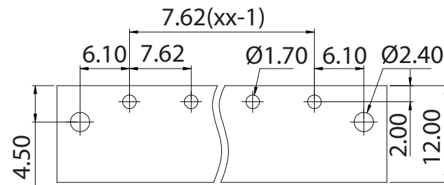
p.c.b. layout
