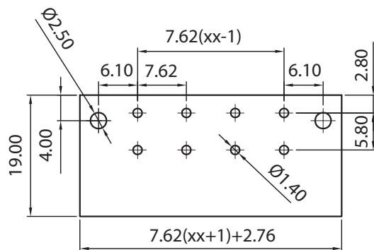
p.c.b. layout
