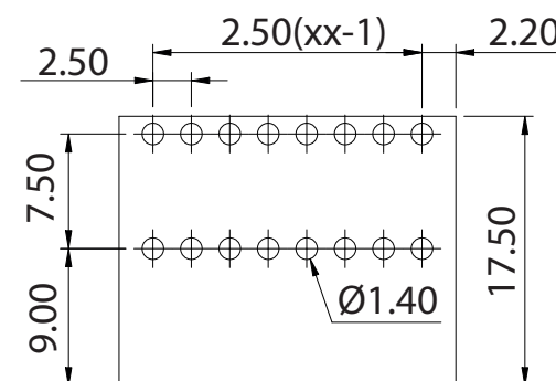
p.c.b. layout
