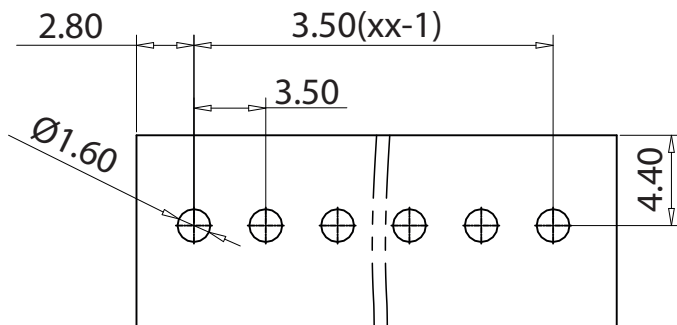
p.c.b. layout
