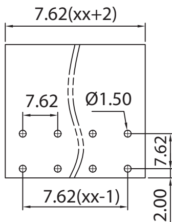
p.c.b. layout
