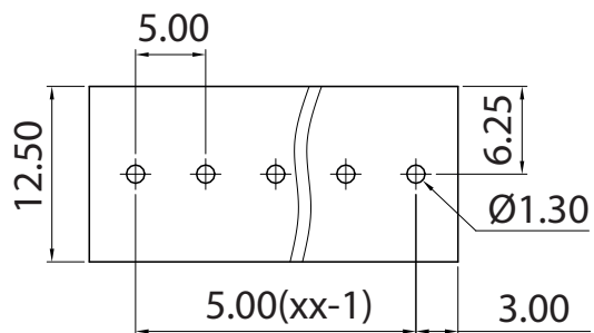
p.c.b. layout
