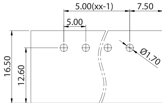
p.c.b. layout
