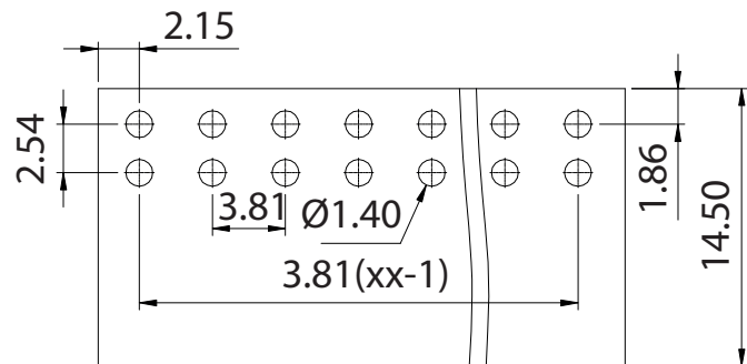
p.c.b. layout
